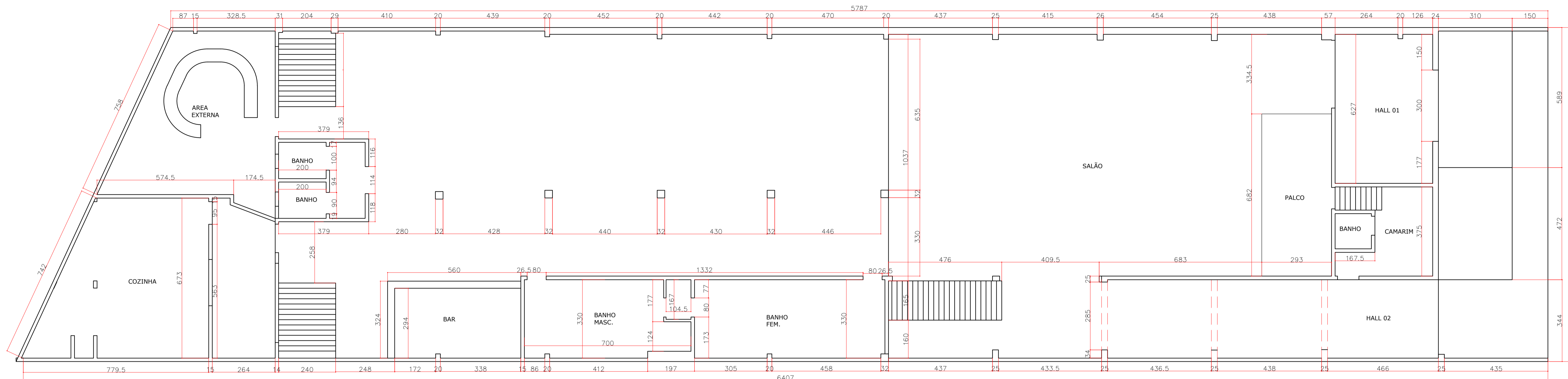
PROJETO BACCUS | PRIMEIRO PAVIMENTO ESCALA 1/100
